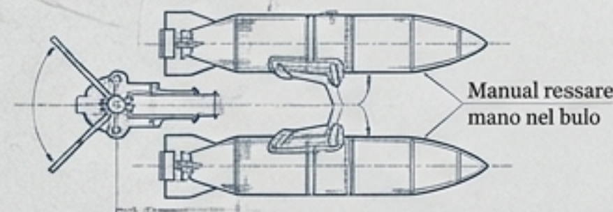
La Mignatta (Siluro di 8 metri, nessuna protezione)
